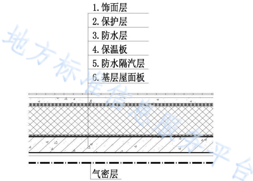
图 3 屋面保温构造做法
