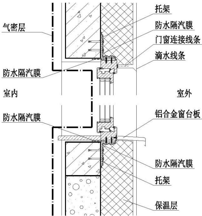
图 6 外窗安装构造做法
